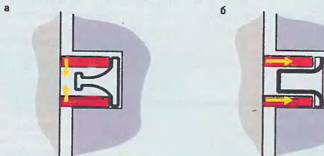
Рис. 2. Самая сложная деталь составного маслосъемного кольца – расширитель. Ему нужно одновременно обеспечить податливость полуколец и необходимое удельное давление на стенку цилиндра. В варианте, показанном на рис. а, обеспечивается изгибная податливость полуколец, здесь расширитель имеет мощную внутреннюю часть (обращенную к цилиндру). Недостаток – подгибание полуколец при работе, истирание их углов и в перспективе – потеря эффективности. В варианте на рис. б полукольца свободны в радиальном направлении, так что отмеченных только что недостатков здесь нет. И все же податливая внутренняя часть расширителя с трудом обеспечивает хорошее прилегание, что со временем тоже приводит к потере эффективности.
