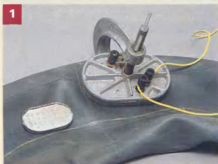
1 Горячий ремонт камер сырой резиной с помощью электровулканизатора или пироставы.
