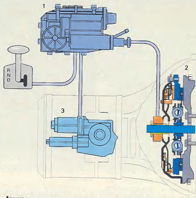
Армия полуавтоматических трансмиссий с каждым днем растет. Компания «Лук» продвигает сразу несколько схем: семейство ASG с электрическими приводами сцепления и переключения передач прижилось на «Опеле-Корсе»: 1 – привод сцепления; 2 – саморегулирующееся сцепление; 3 – привод коробки передач.
