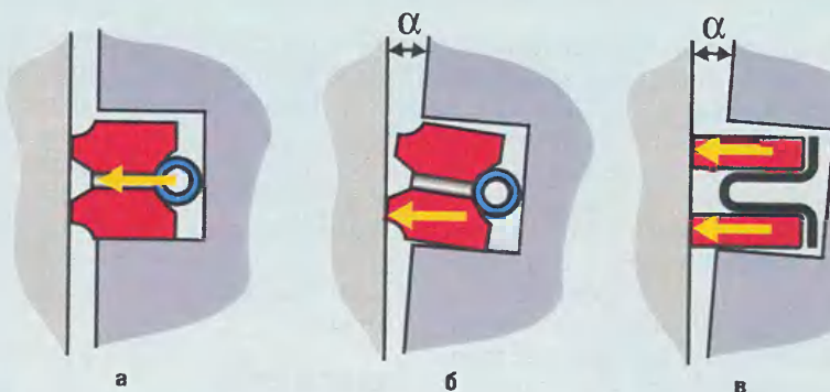
Рис. 1. Один из недостатков маслосъемного кольца коромыслового типа (а): при перекладке поршня или под действием иных факторов оно начинает работать лишь частью своей поверхности (б), что ухудшает снятие масла с зеркала цилиндра и приводит к повышенному износу. Подобное наиболее заметно в двигателях со значительным износом деталей цилиндропоршневой группы. Составное кольцо при этом продолжает нормально работать, поскольку его нижняя и верхняя части независимы друг от друга (в).
