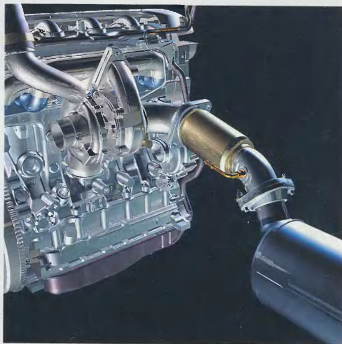
Новый фильтр длиной 150–300 мм устанавливают рядом с выпускным коллектором (двигатель «Рено» 2,2 л).
