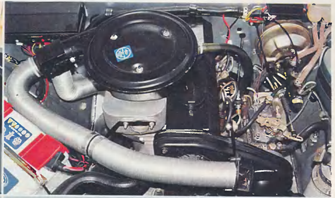
Под капотом «Сталкера» дизель ВАЗ-341.
