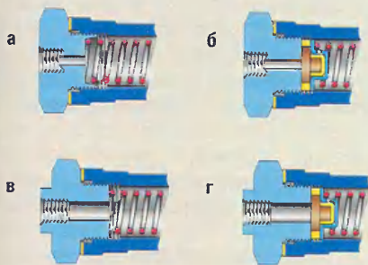
Рис. 2. Похожие, но разные: а – главный цилиндр привода сцепления, дет. 408-1609010 («Москвич-408»); б – главный цилиндр привода сцепления, дет. 4301-1602290 (ГАЗ моделей 24-10, 31029, 3110, 3102, 53 и т. п.); в – главный цилиндр привода сцепления, дет. 24-1602300 (ГАЗ-24); г – главный тормозной цилиндр, дет. 408-3505010 («Москвич-408»).
