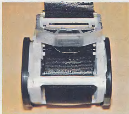
Ремень безопасности с механическим фиксатором – грабером.
