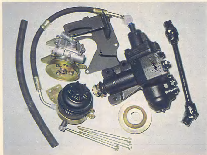
Установочный комплект гидроусилителя руля ГУР 21.3400012 снабжен подробной инструкцией, и монтаж его на автомобиль по силам даже новичку.
